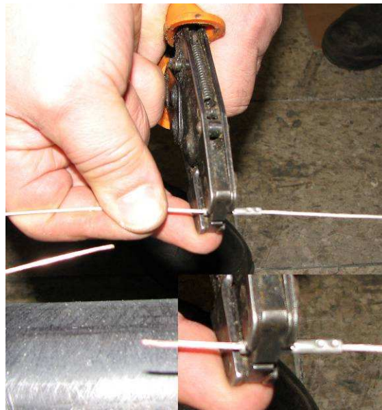
Unir los cables de detección utilizando una tenaza de apriete
