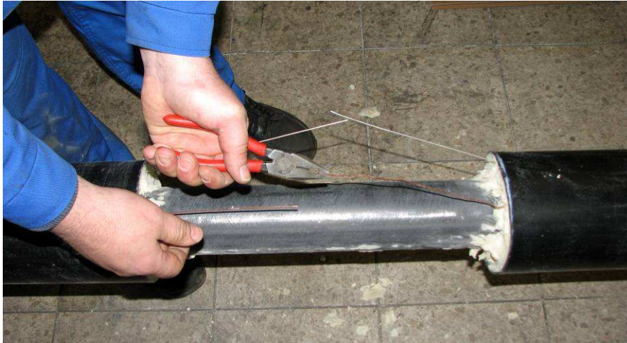
Prueba de tracción de los cables de detección
