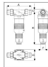
Gráfico: Medidas JSY-LF-A 1 ½"-2"
