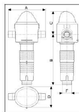
Gráfico: Medidas JSY-LF-A ¾"-1 ¼"
